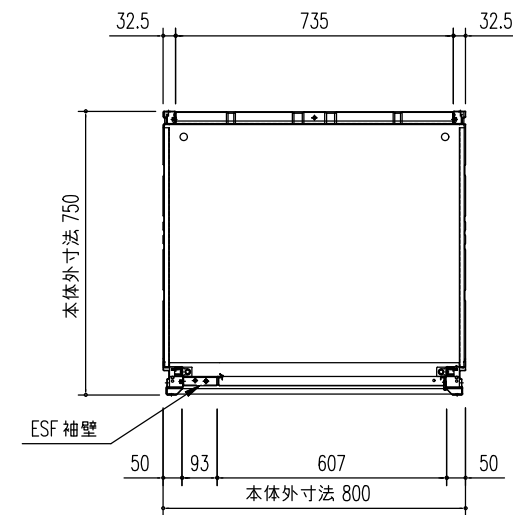
平面図 (S=1/20)
