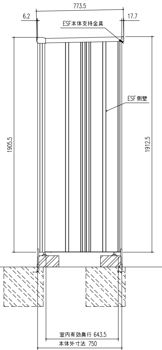
側面図 (S=1/20)
