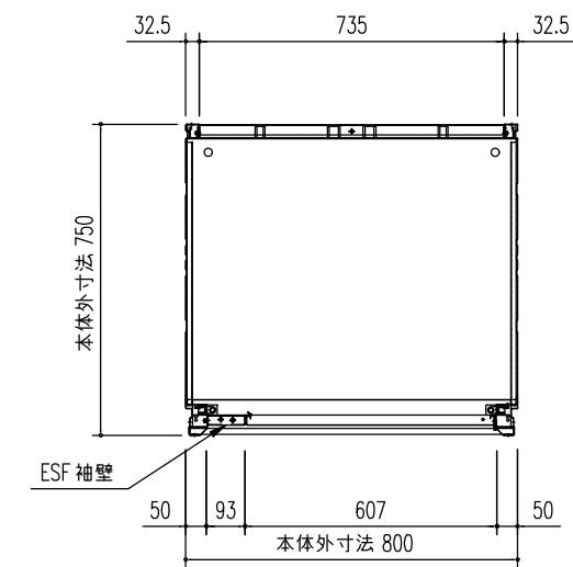
平面図 (S=1/20)
