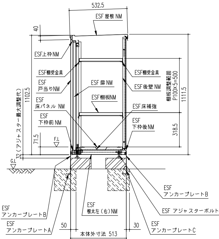
矩計図 (S=1/20)
