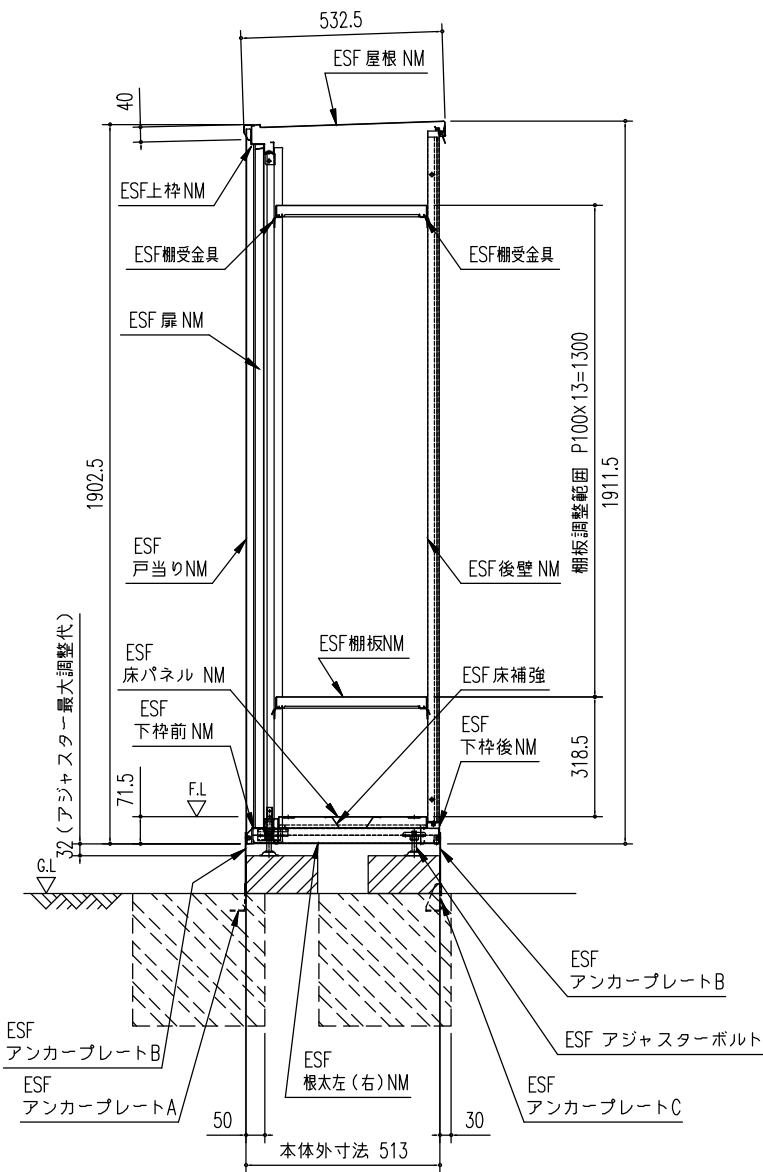
矩計図 (S=1/20)
