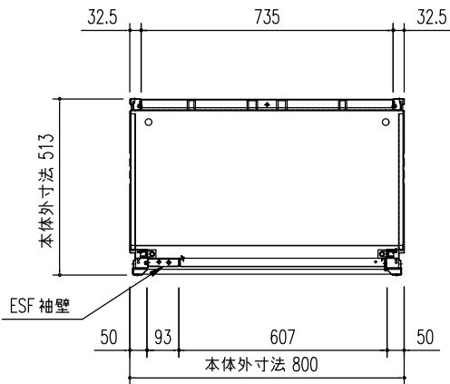
平面図 (S=1/20)
