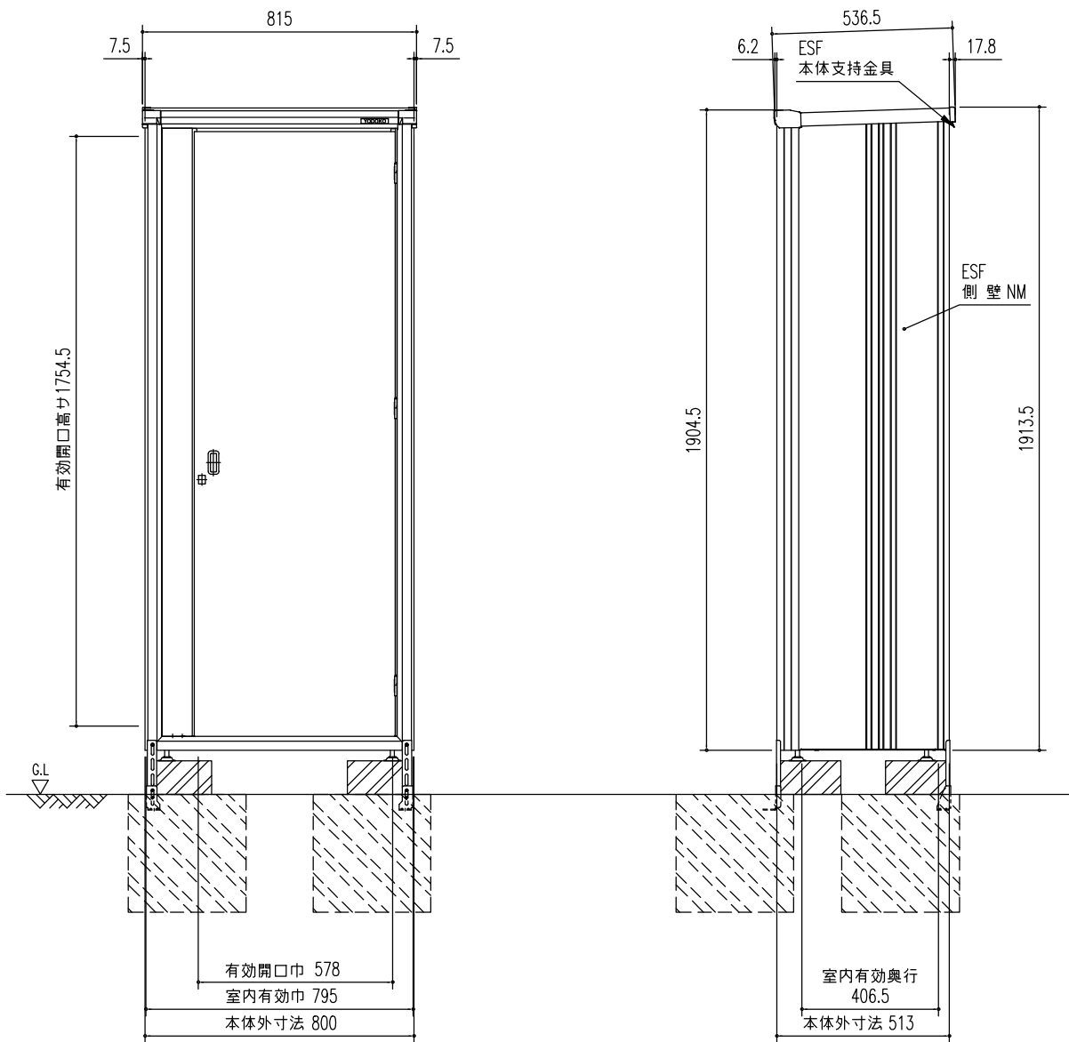
正面立面図 (S=1/20)
