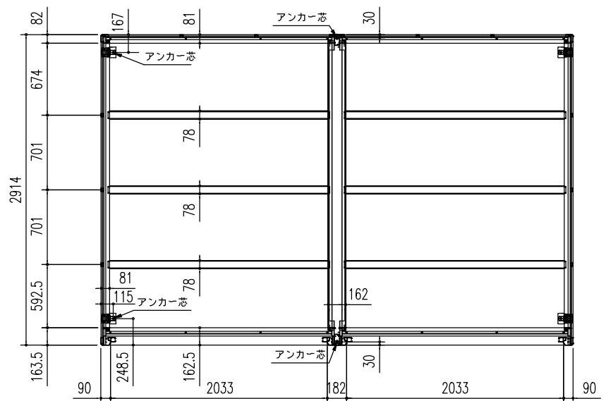
床伏図 (S=1/50)
