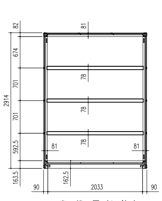
床伏図 (S = 1/50)
