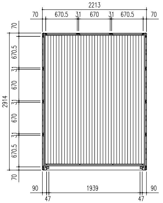
平面図 (S = 1/50)
