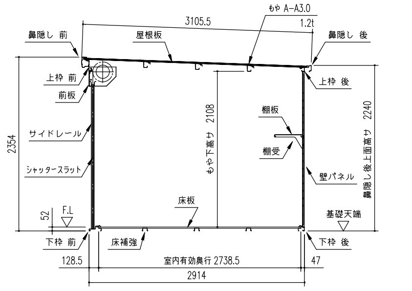
一般型矩計図 (S = 1/50)
