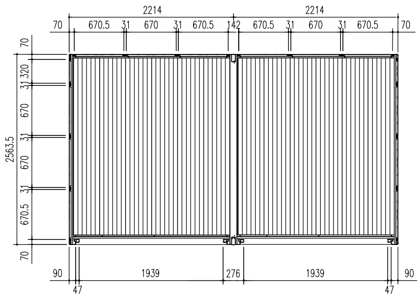
平面図 (S = 1/50)
