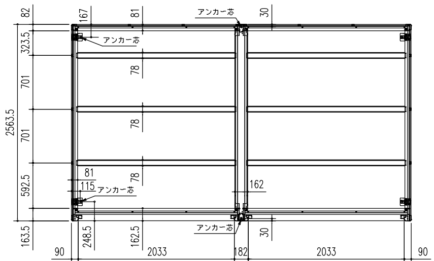
床伏図 (S = 1/50)
