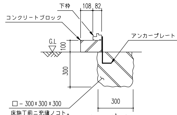
A ~ A' 断面 (外アンカー用) ブロック基礎断面図例 (S = 1/20)
