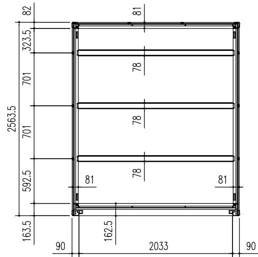
床伏図 (S = 1/50)
