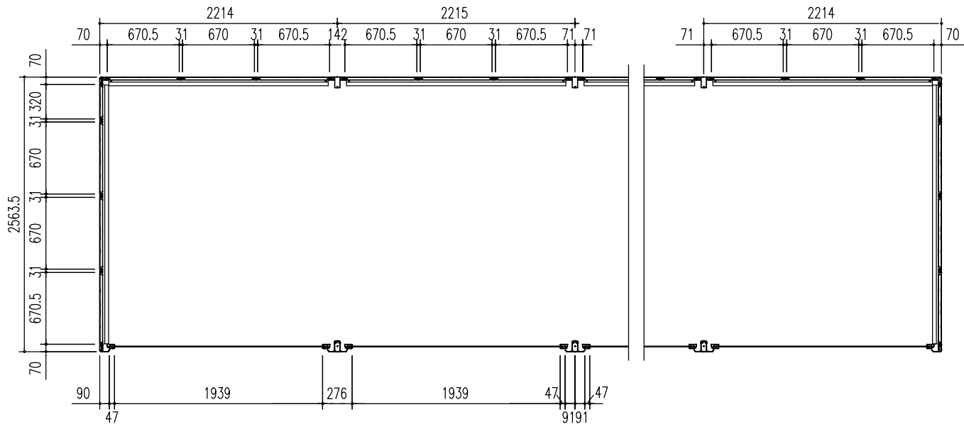
平面図 (S = 1/50)
