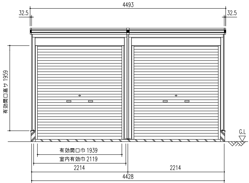
正面立面図 (S = 1/50)
