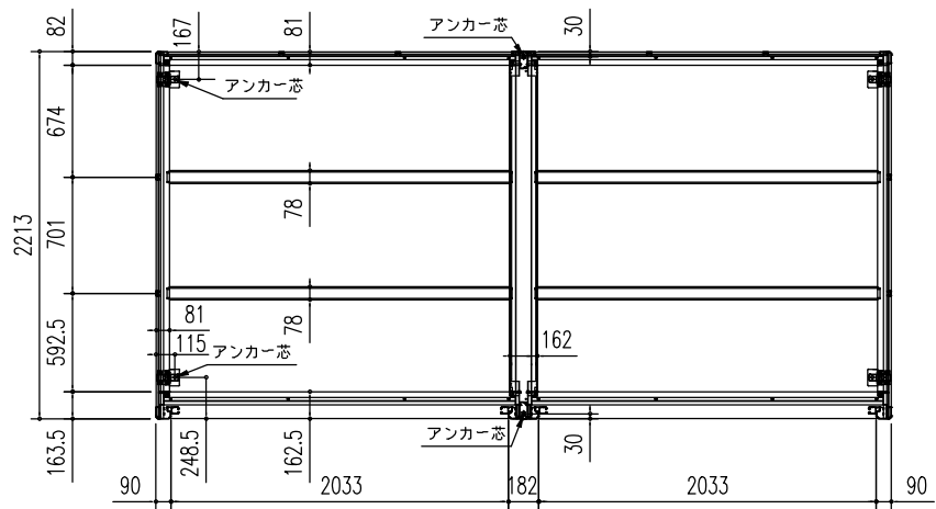
床伏図 (S= 1/50)
