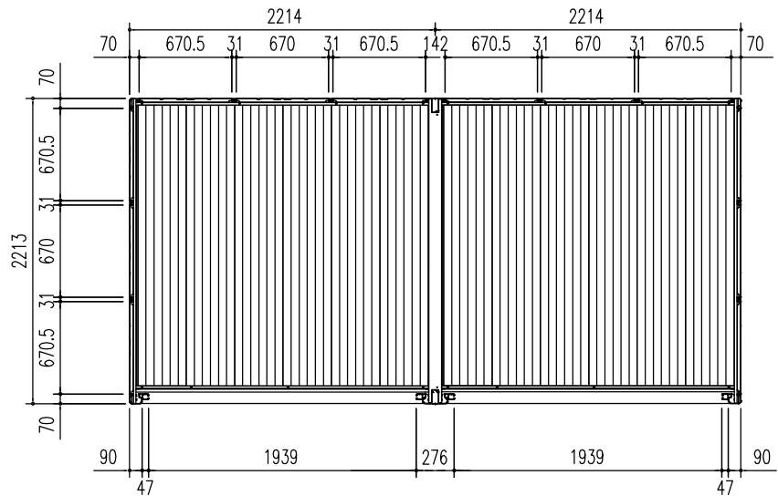
平面図 (S= 1/50)
