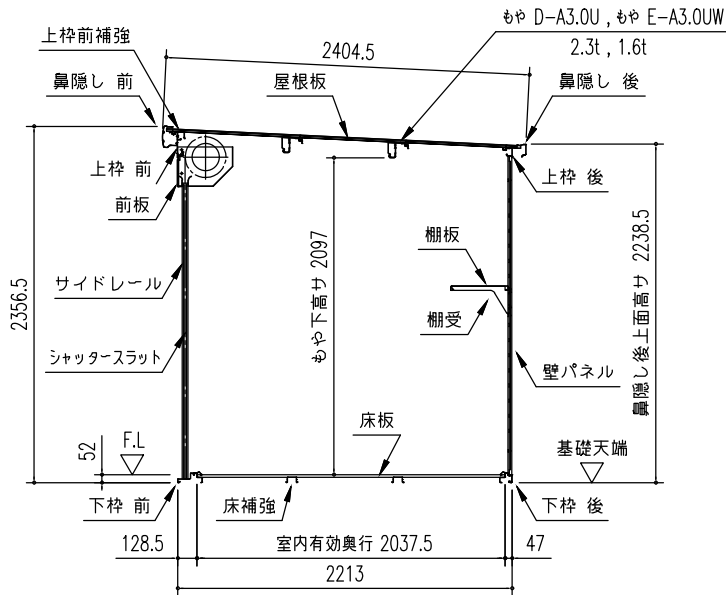
豪雪型矩計図 (S= 1/50)
