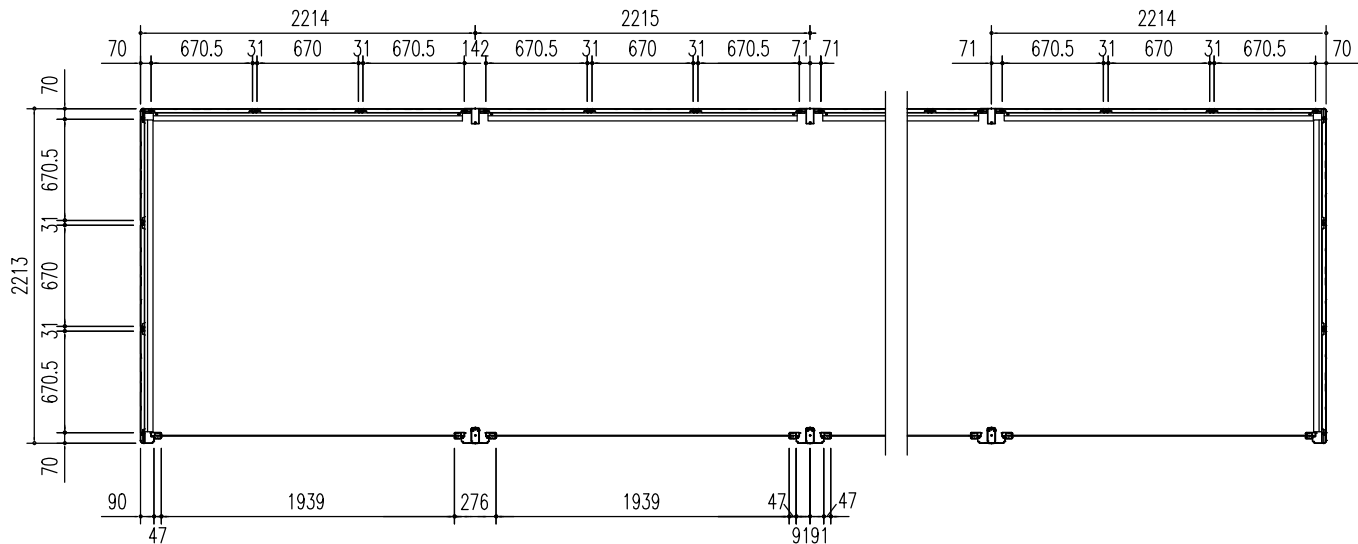
平面図 (S = 1/50)
