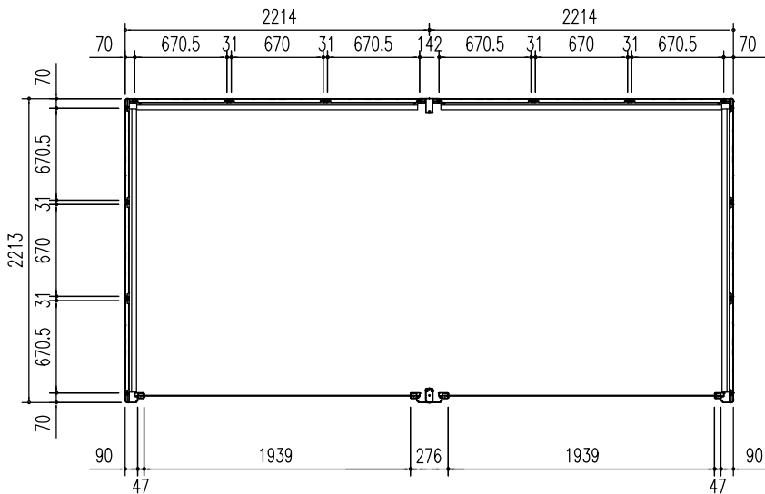
平面図 (S = 1/50)
