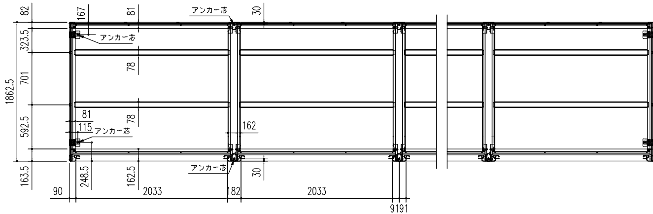
床伏図 (S = 1/50)
