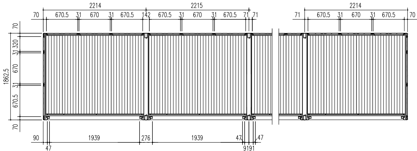
平面図 (S = 1/50)
