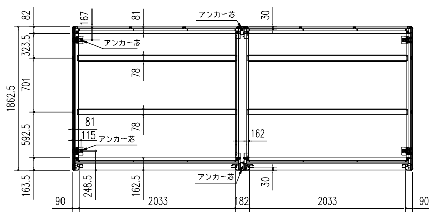
床伏図 (S = 1/50)
