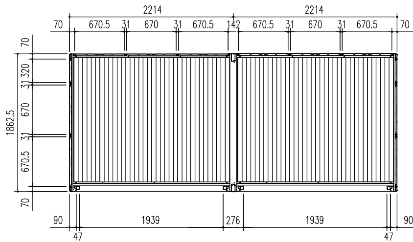
平面図 (S = 1/50)
