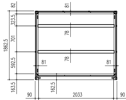
床伏図 (S=1/50)
