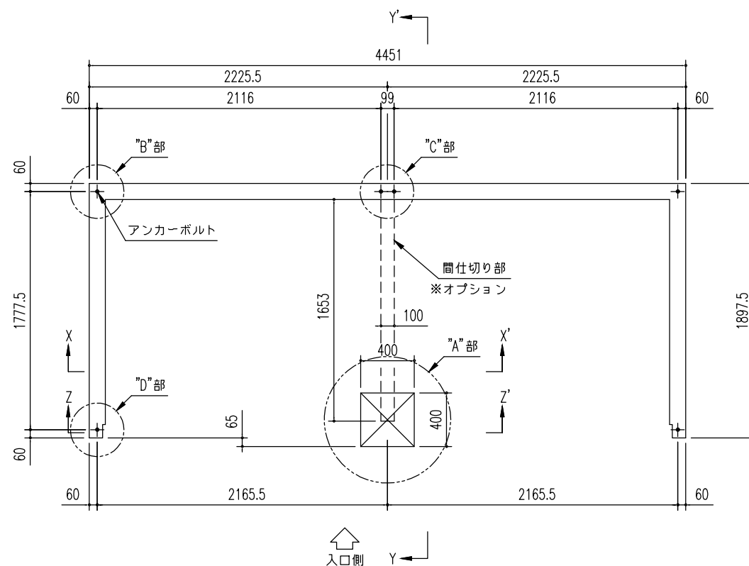
基礎伏図 (S=1/40)
