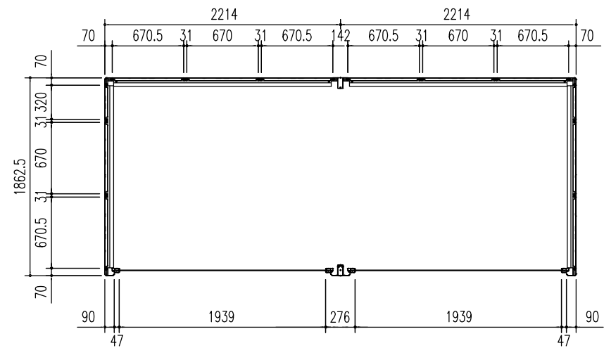
平面図 (S = 1/50)
