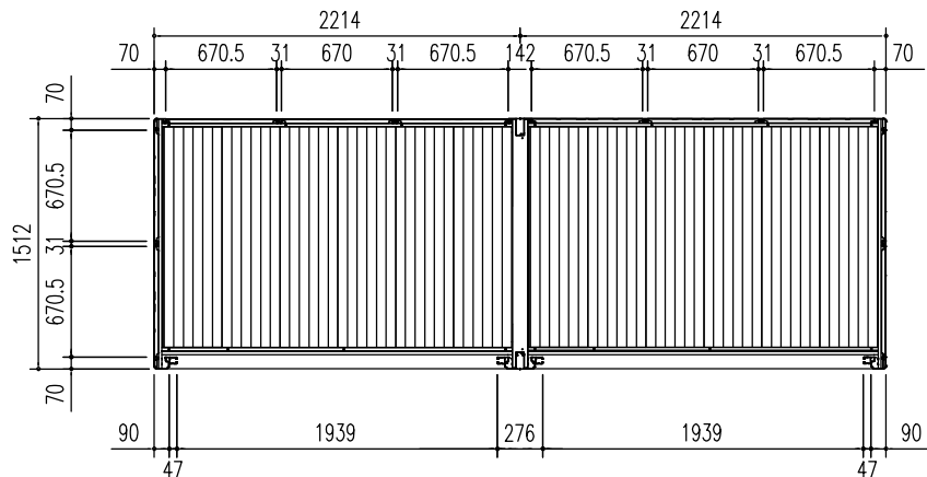
平面図 (S = 1/50)
