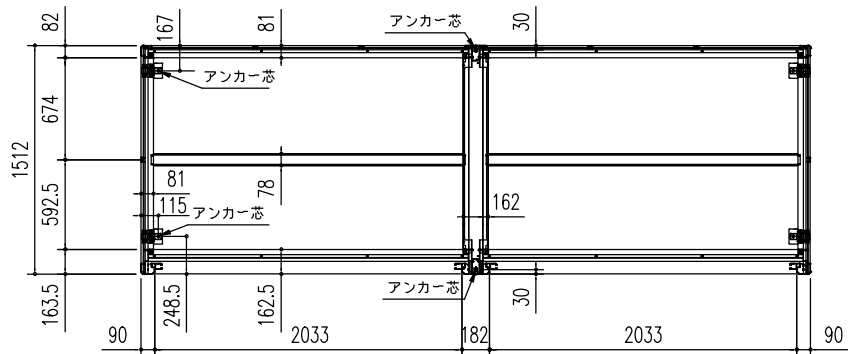
床伏図 (S = 1/50)
