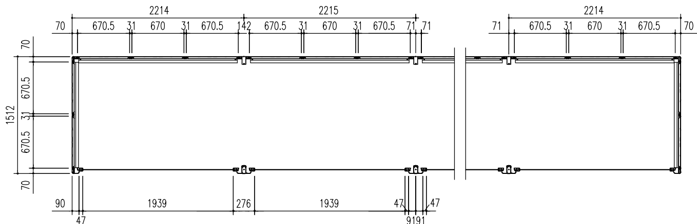
平面図 (S = 1/50)
