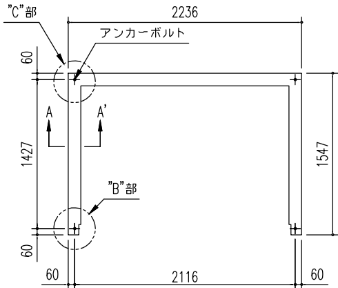
布基礎伏図 (S=1/50)
