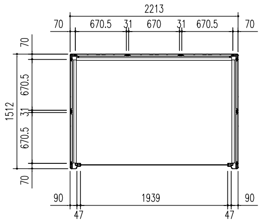
平面図 (S=1/50)
