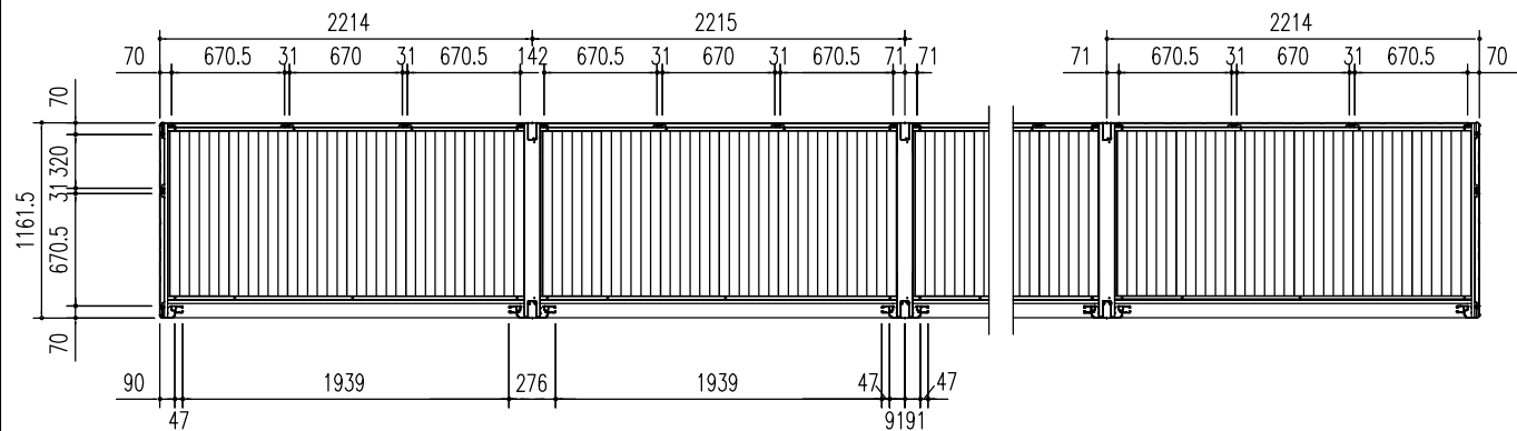
平面図 (S = 1/50)
