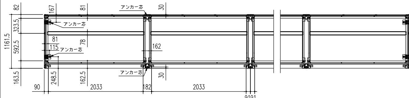
床伏図 (S = 1/50)
