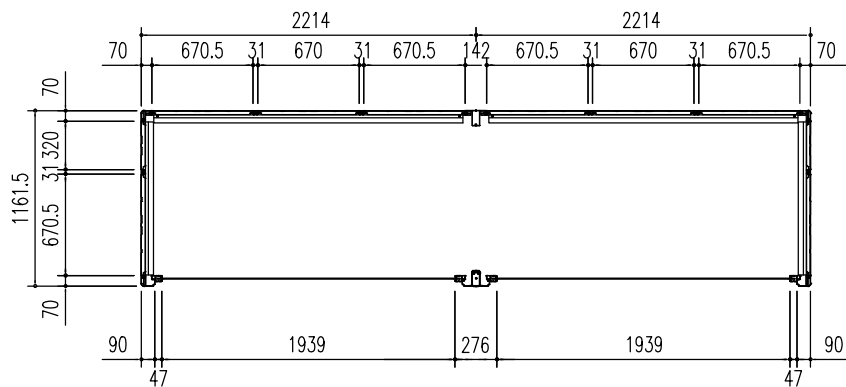
平面図 (S = 1/50)
