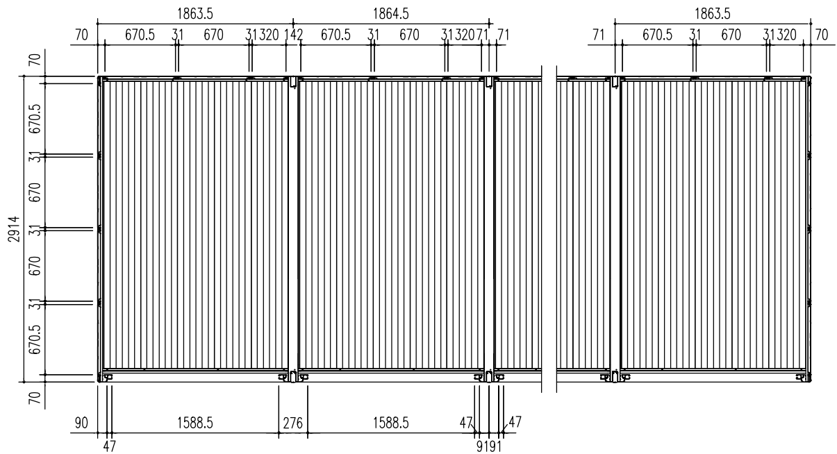
平面図 (S = 1/50)
