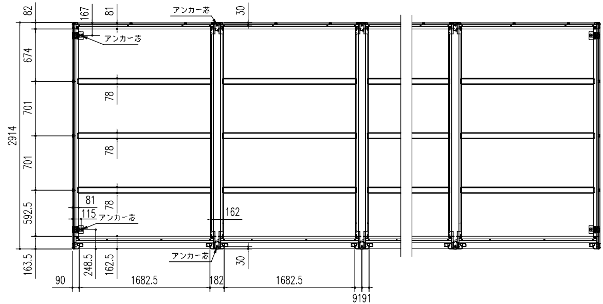
床伏図 (S = 1/50)
