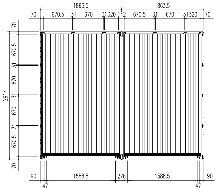
平面図 (S = 1/50)
