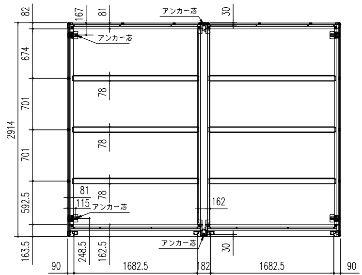
床伏図 (S = 1/50)
