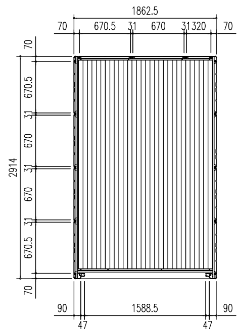
平面圖 (S = 1/50)
