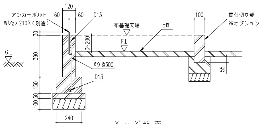
X ~ X'断面 基礎断面図 (S=1/20)
