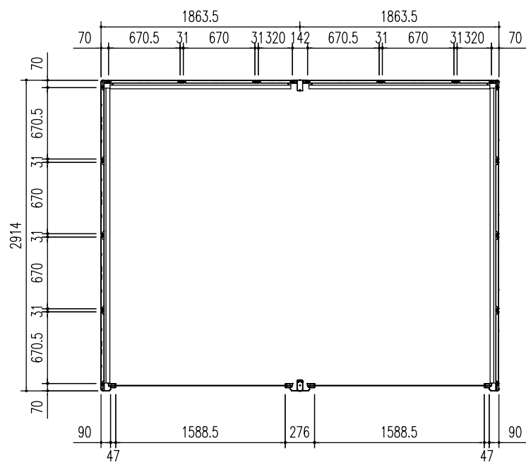
平面図 (S = 1/50)
