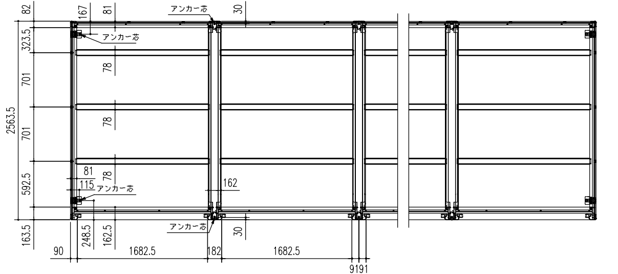
床伏図 (S = 1/50)
