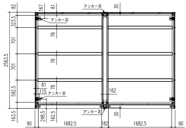
床伏図 (S = 1/50)
