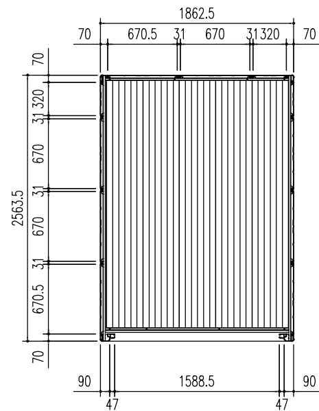
平面图 (S = 1/50)
