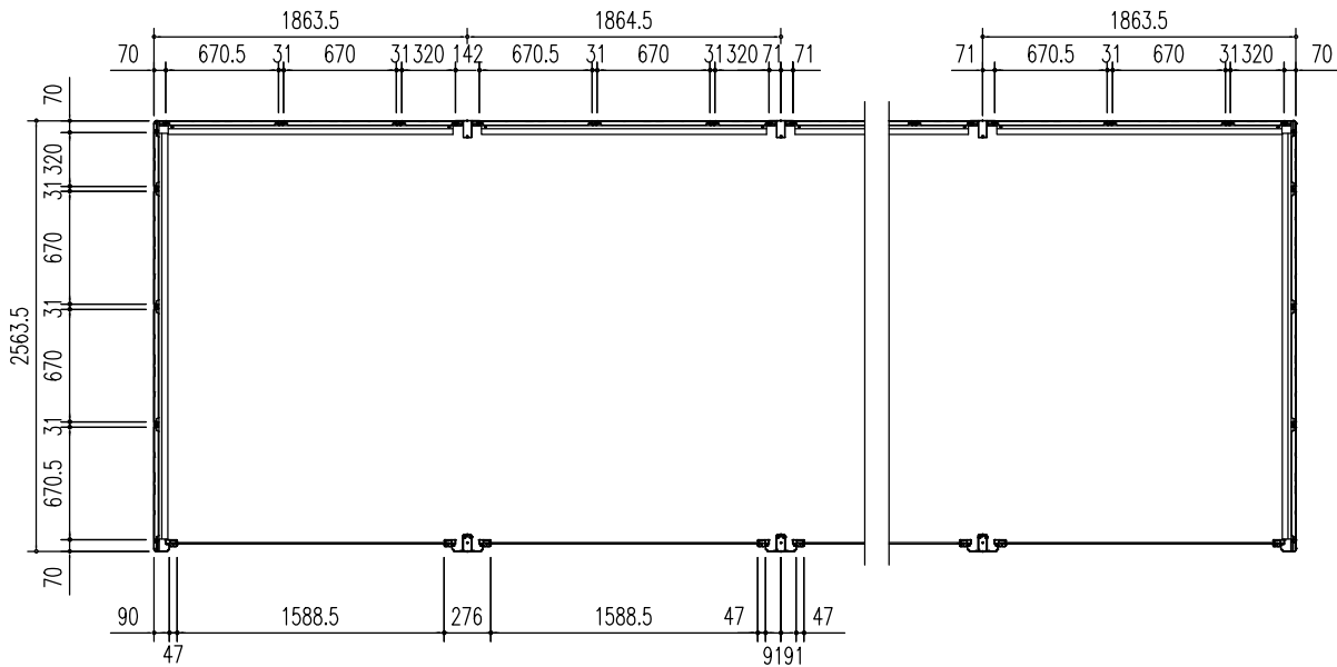
平面図 (S = 1/50)
