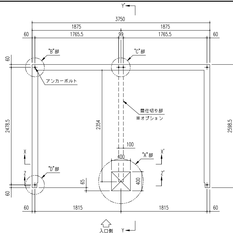
基礎伏図 (S=1/40)
