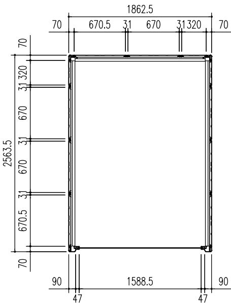
平面図 (S=1/50)
