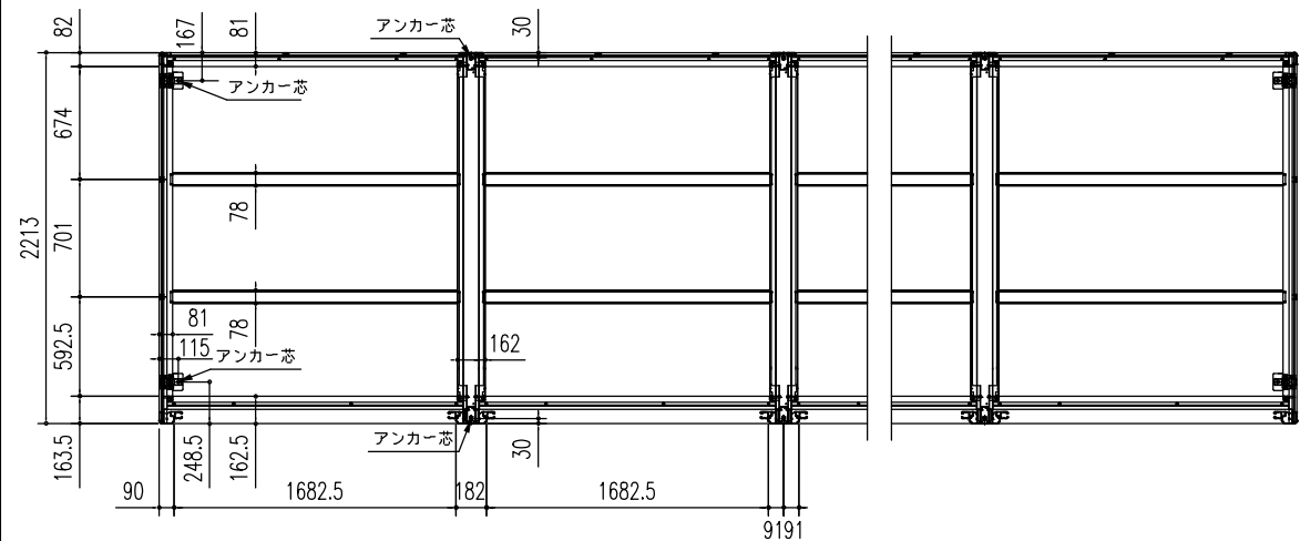
床伏図 (S = 1/50)
