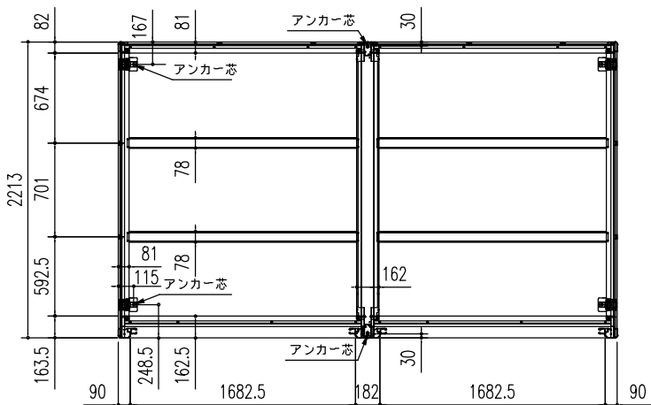
床伏図 (S = 1/50)
