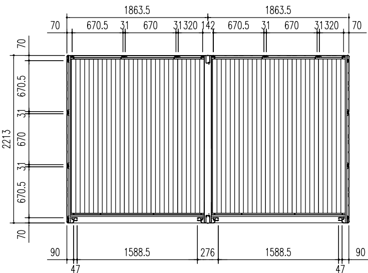
平面図 (S = 1/50)
