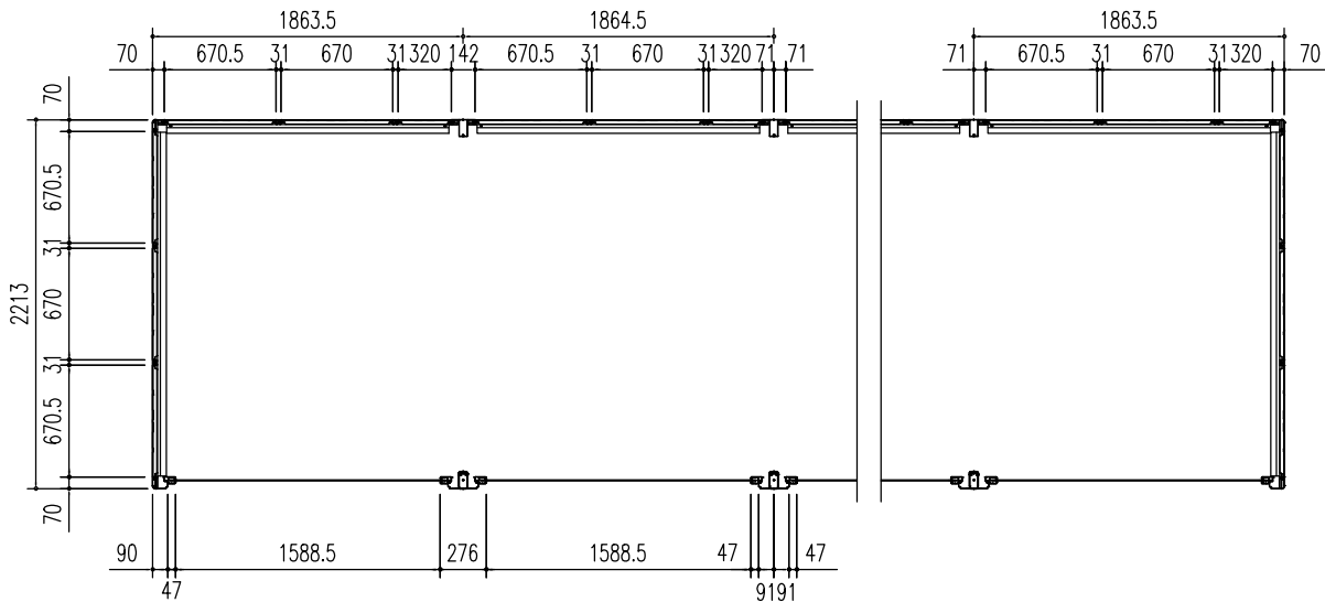
平面図 (S = 1/50)
