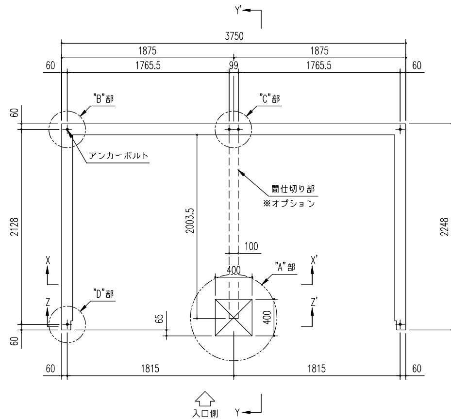
基礎伏図 (S=1/40)
