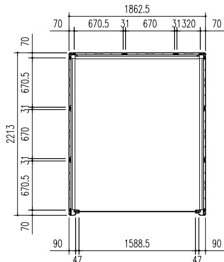
平面図 (S=1/50)
