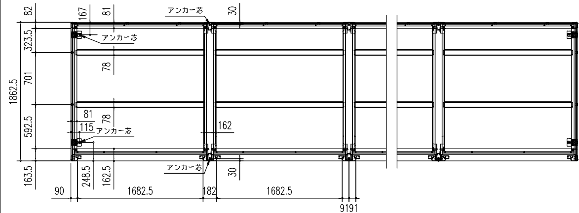
床伏図 (S = 1/50)
