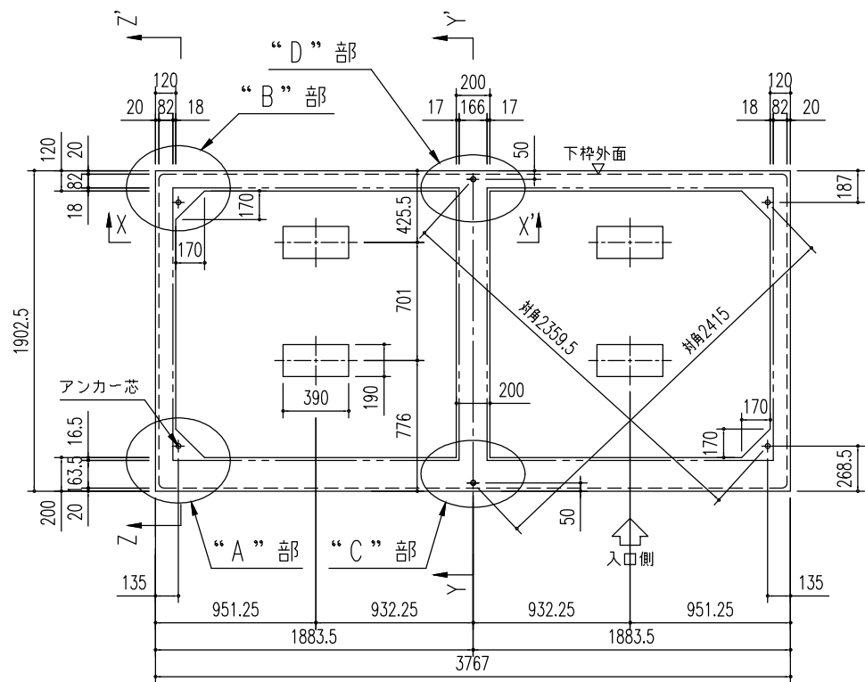
基礎伏図 (S=1/40)
