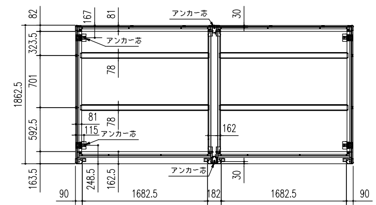
床伏図 (S = 1/50)
