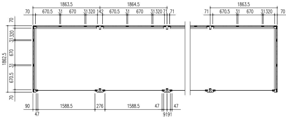
平面図 (S = 1/50)
