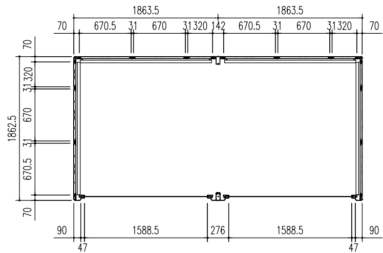
平面図 (S = 1/50)
