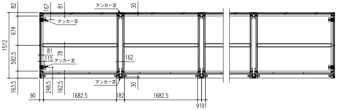
床伏図 (S = 1/50)
