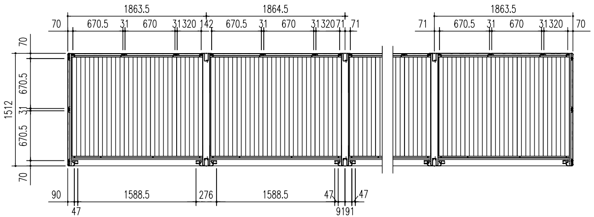
平面図 (S = 1/50)
