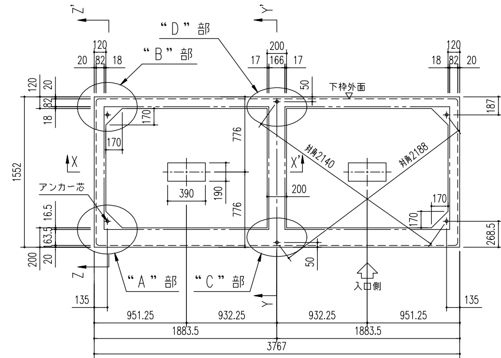
基礎伏図 (S=1/40)
