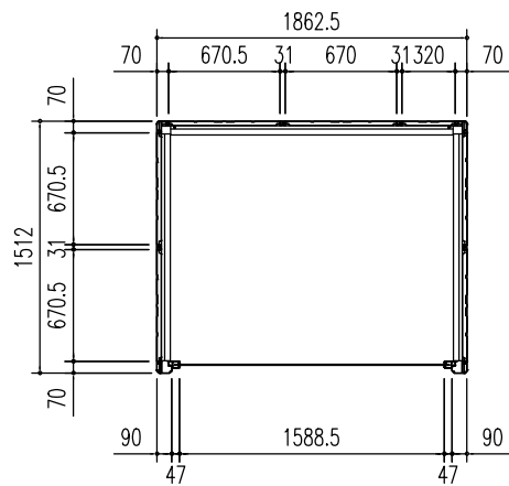
平面図 (S=1/50)
