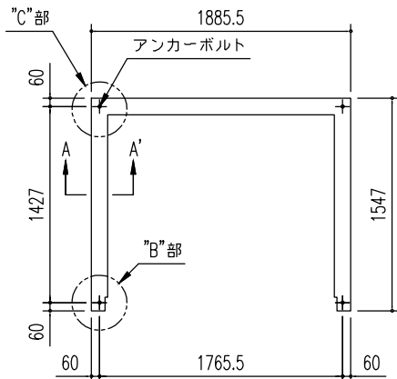
布基礎伏図 (S=1/50)
