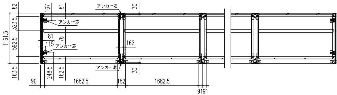
床伏図 (S = 1/50)
