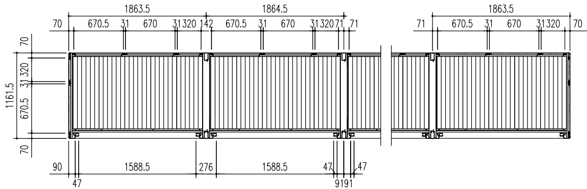
平面図 (S = 1/50)
