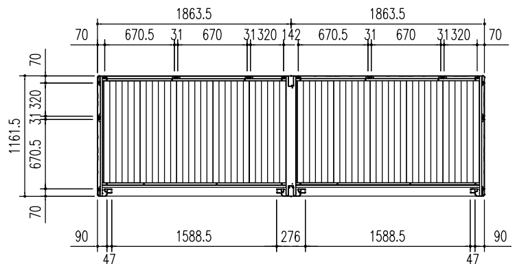
平面図 (S = 1/50)
