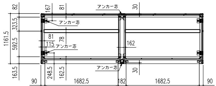
床伏図 (S = 1/50)
