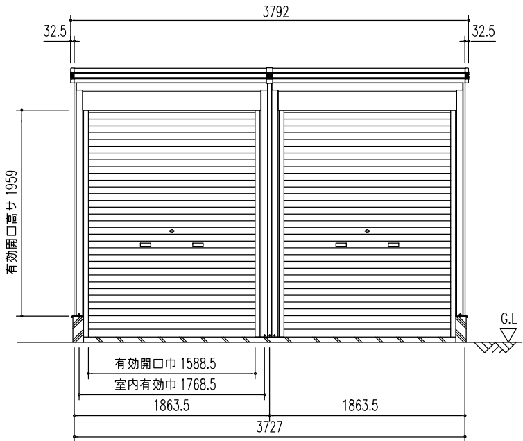
正面立面図 (S = 1/50)
