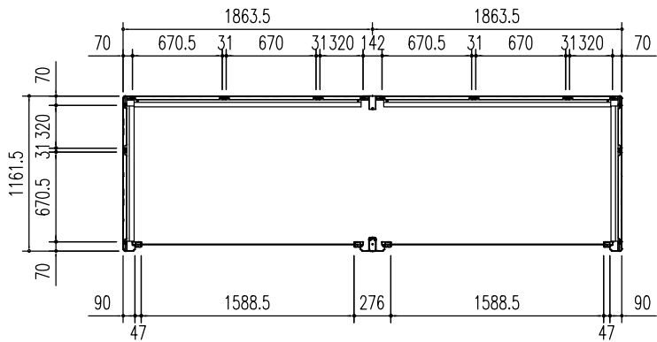
平面図 (S = 1/50)
